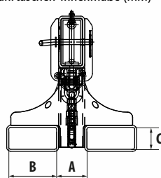
Einfahrtaschen-Innenmaße (mm)
